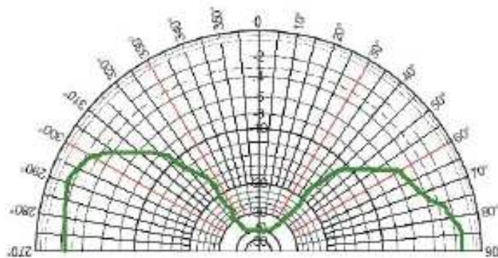
Elevation Pattern (Z, Y or H-Plane)
