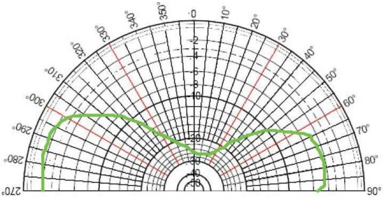
Elevation Pattern (Z, Y or H-Plane)
