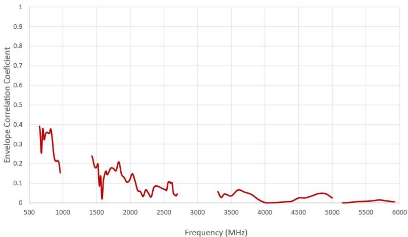
Coefficient de corrélation de l'enveloppe câble 2 et 3
