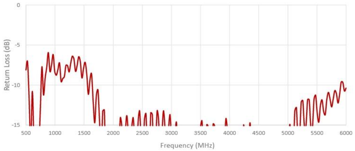
Cable 4: 5GNR
