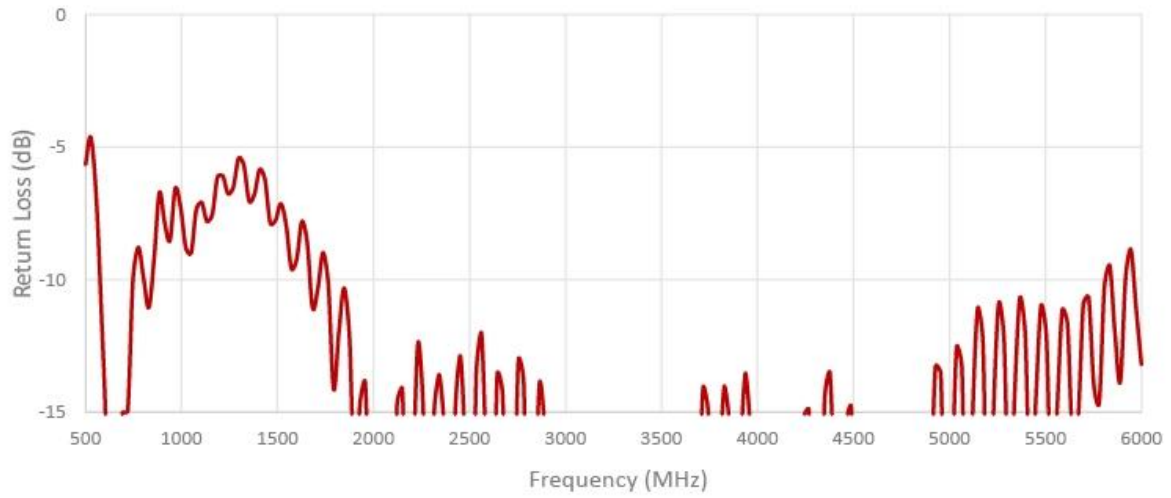
Cable 3: 5GNR
