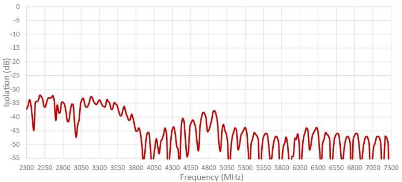
Isolation câble 5 et 7
