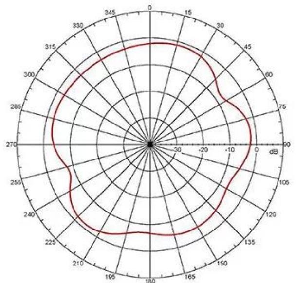
H-Plane
